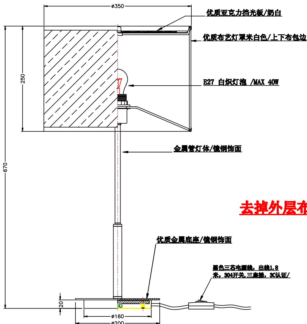
主视图
